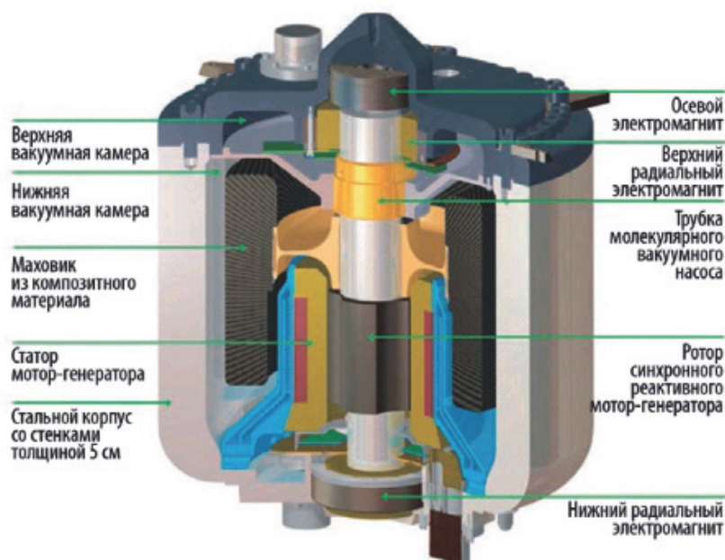
Рисунок 1 – Конструкция супермаховика
