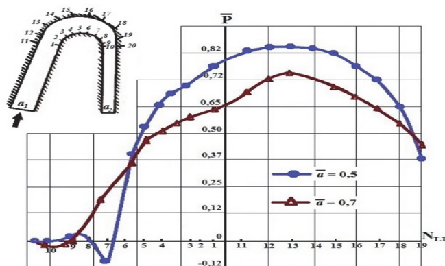
Рисунок 4 – Изменение относительного давления на стенках каналов при различной конфузурности
