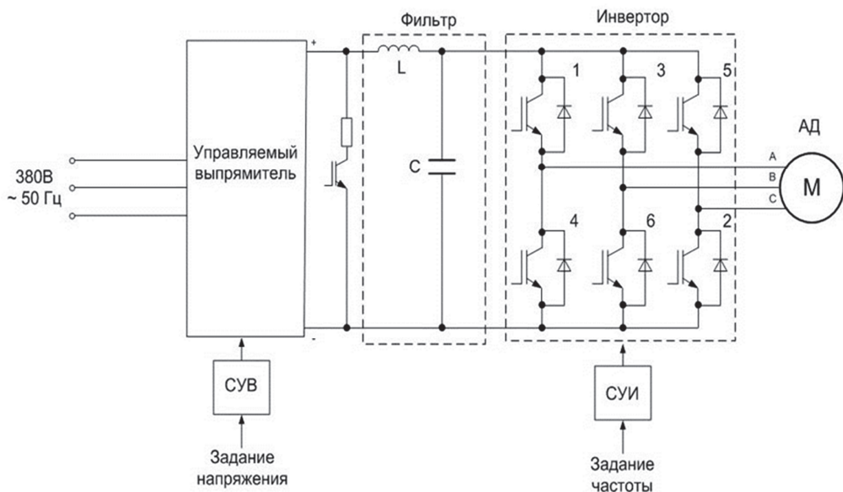
Рисунок 1 – Преобразователь частоты
