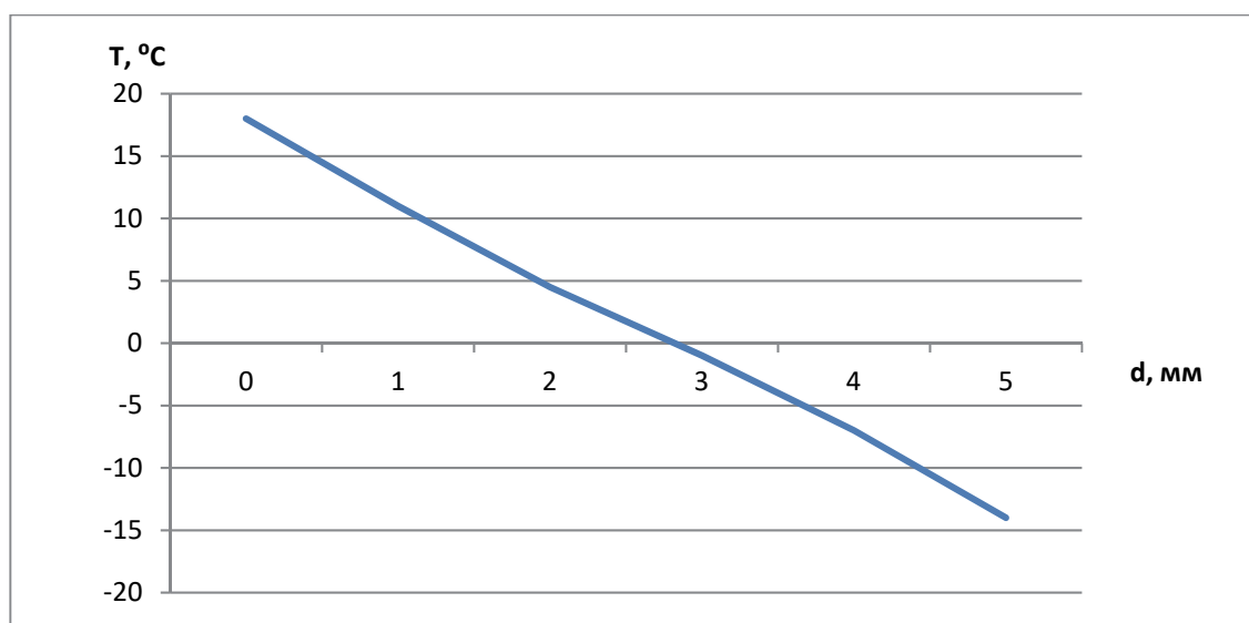
Рисунок 2 – График зависимости температуры от толщины стенки
