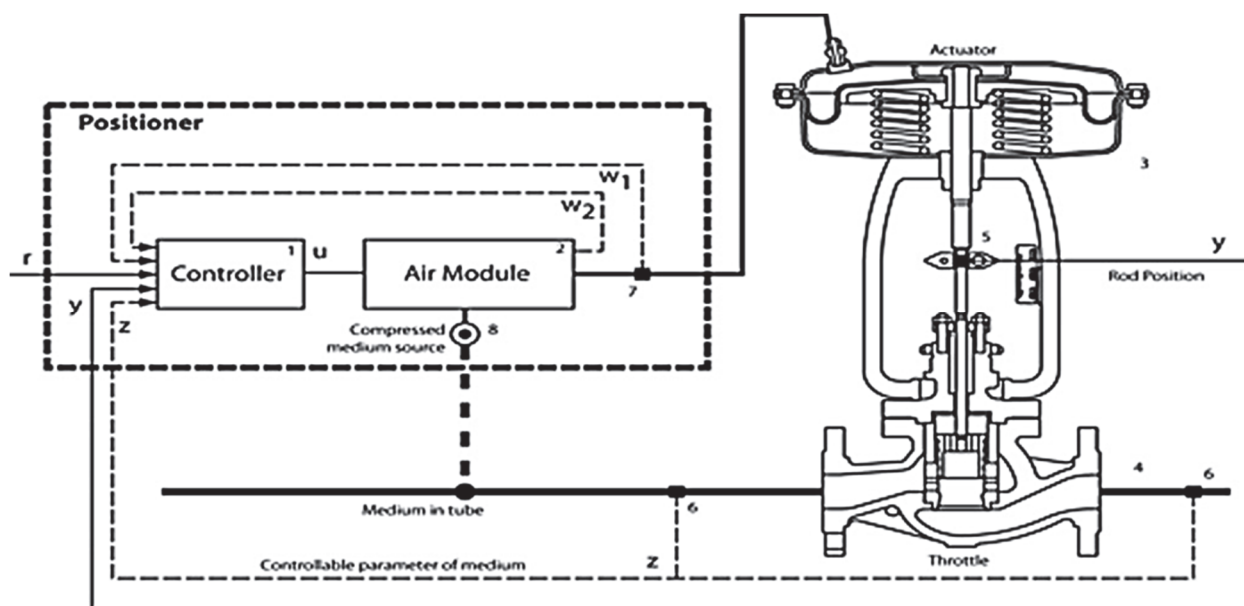
Рисунок 1 – Схема работы системы управления трубопроводным клапаном: 1 – контроллер; 2 – воздушный модуль; 3 – пневмопривод; 4 – дроссельная заслонка; 5 – датчик положения; 6 – датчики параметров; 7 – дополнительные датчики состояния привода; 8 – источник подачи воздуха
