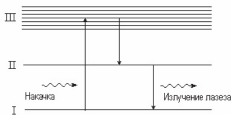
Рисунок 2 – Схема энергетических уровней трёхуровневого лазера
