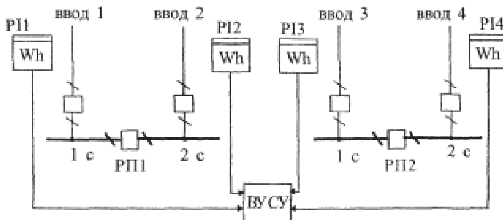
Рисунок 1 – Принципиальная схема автоматизированного учета электроэнергии
