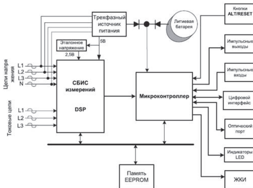
Рисунок 5 – Структурная схема многофункционального счетчика Альфа А1Т
