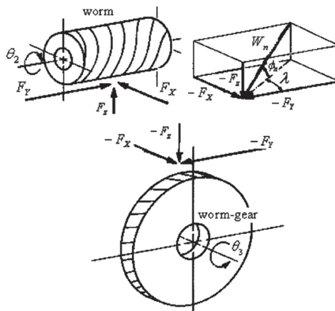
Рисунок 2 – Разложение контактных сил
