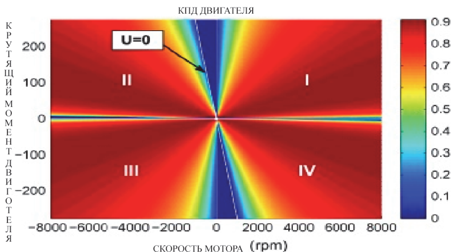
Рисунок 2 – График контура КПД двигателя для двигателя
